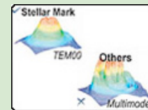
TEM00 Strahlmodus
